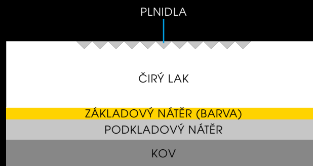
VADA OPRAVENÁ PASTOU S PLNIDLEM
