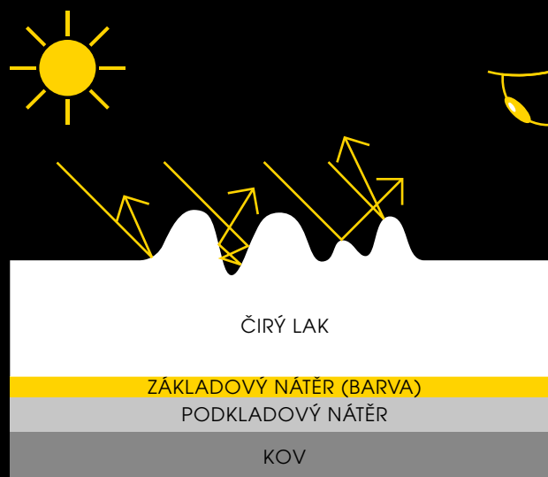
POVRCHOVÉ VADY MAJÍ NEGATIVNÍ ÚČINEK VIDITELNÉ NA SVĚTLE
